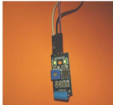
Gambar 4. Sensor Getar Kasur Pasien
